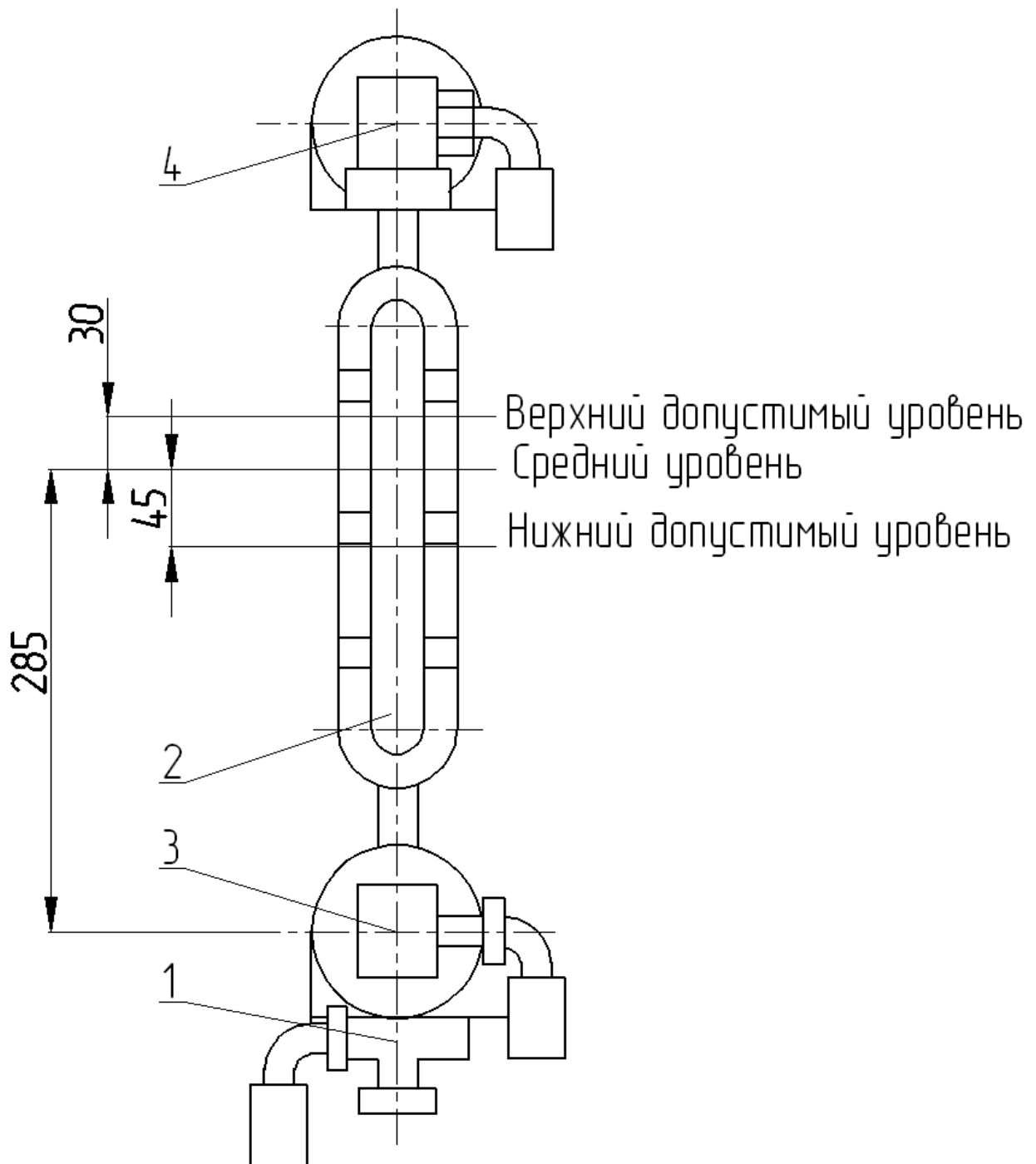
Рис. 3 Водоуказательный прибор.
