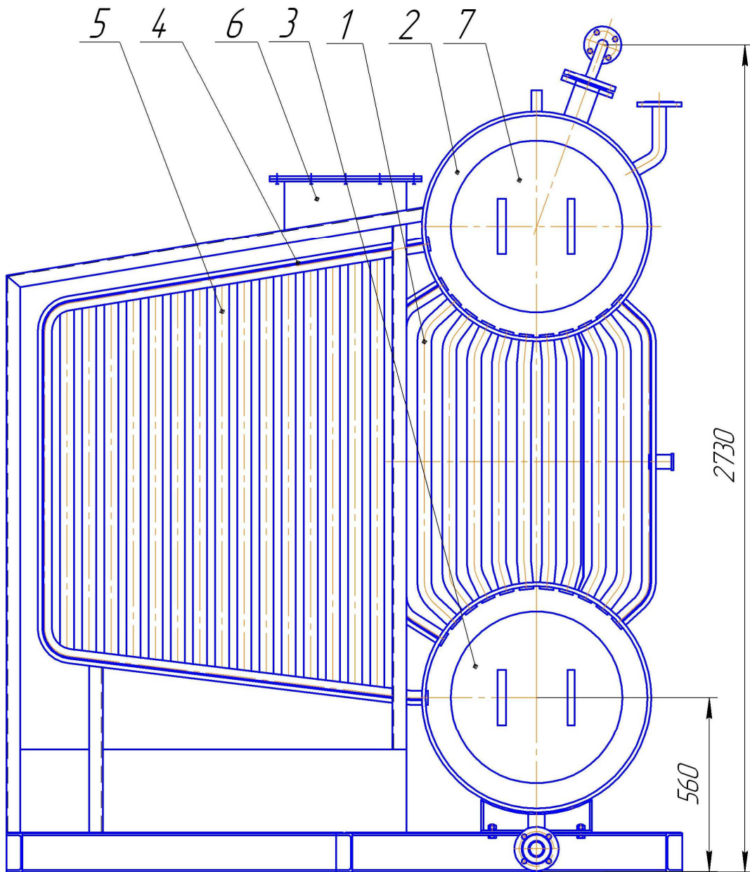
Рис.2 Система трубная
