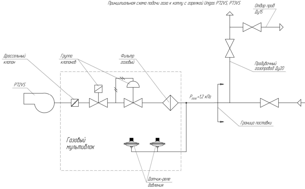
Принципиальная схема подачи газа к котлу с горелкой Unigas P72VS, P73VS
