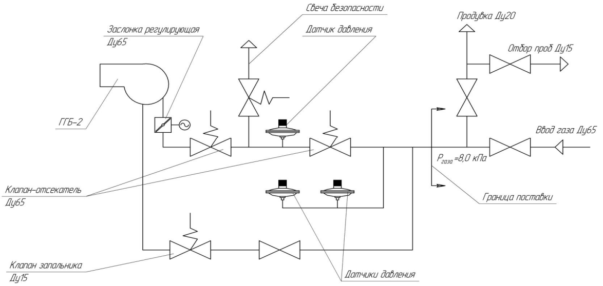
Принципиальная схема подачи газа к котлу с горелкой ГТБ-2
