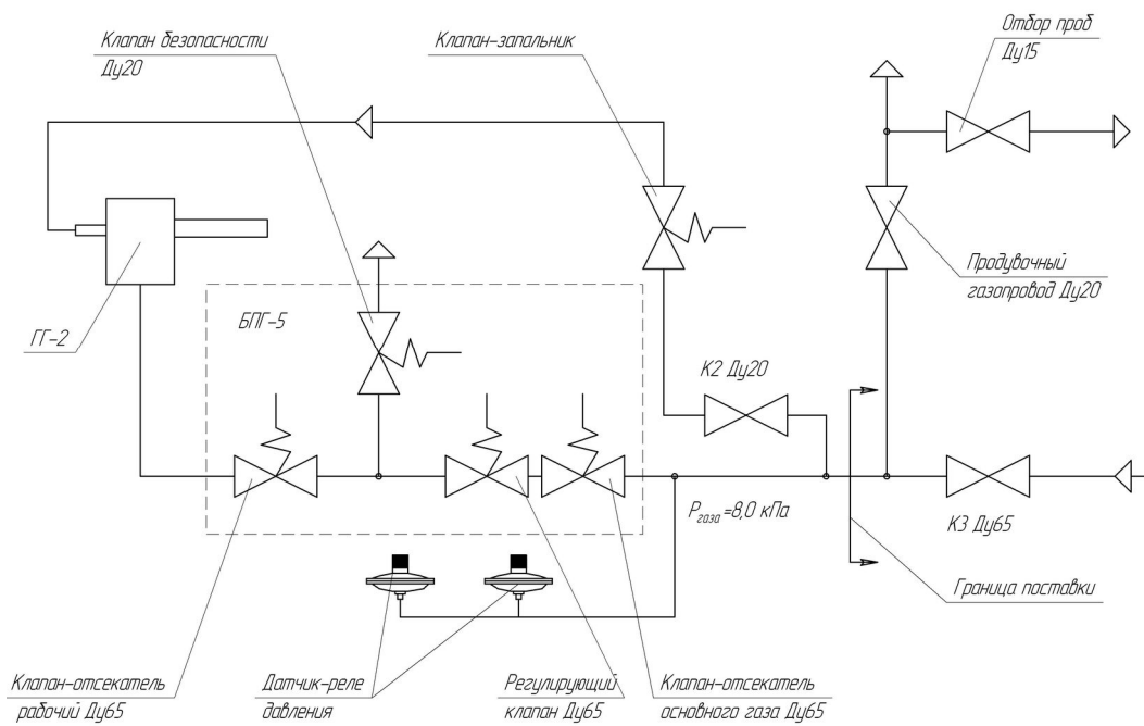
Принципиальная схема подачи газа к котлу с горелкой ГГ-2
