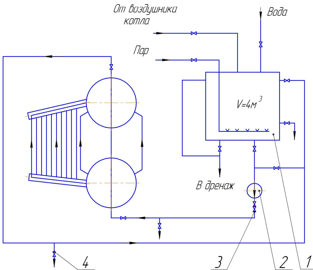
Рис.4 Котел
