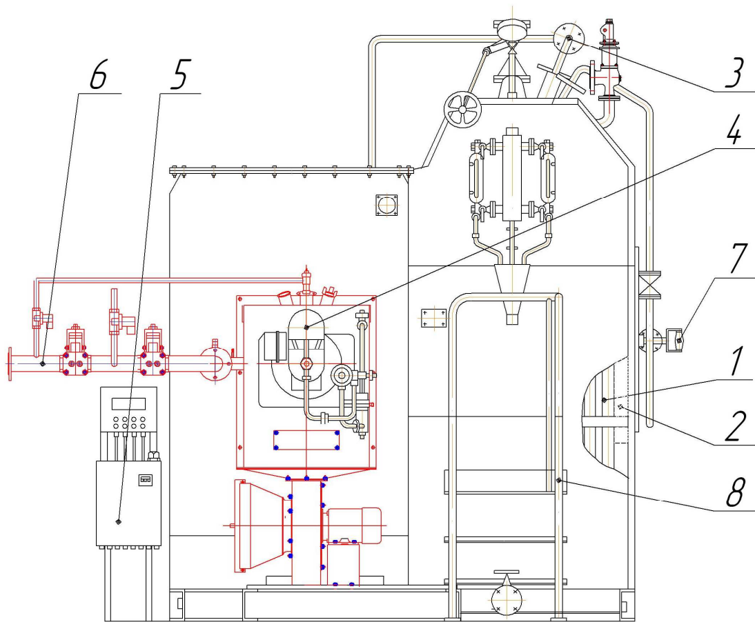
Рис.1 Котел паровой
