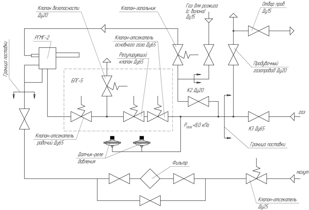
Принципиальная схема подачи топлива к котлу с горелкой РГМГ-2
