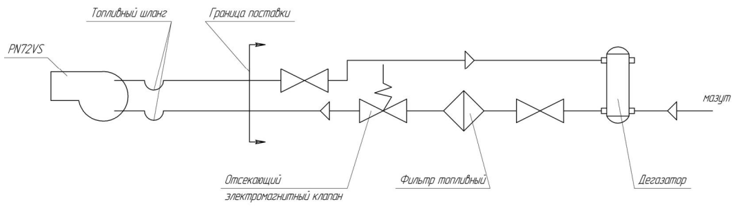
Принципиальная схема подачи топлива к котлу с горелкой Unigas PN72VS, PN81VS
